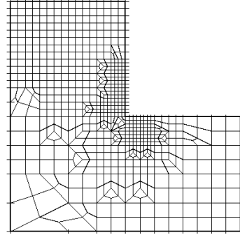
Fig. 24. Resulting mesh
