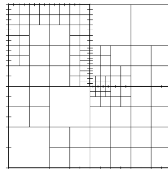
Fig. 17. Initial quadtree
