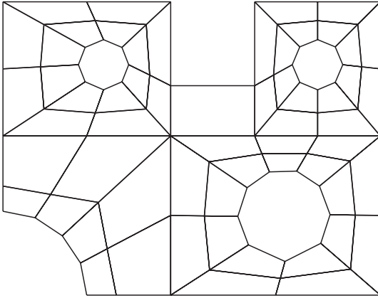
Fig. 49. Initial finite element mesh (Q4)
